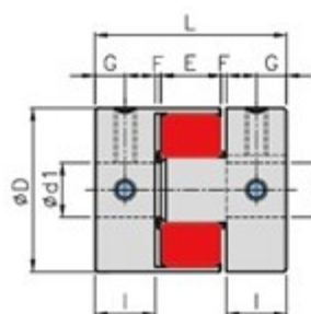
TYPE : SRJ-20-RD ~ SRJ-30-RD
