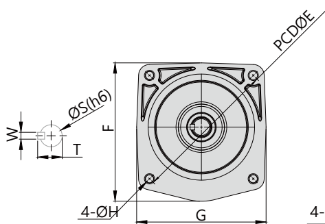
A型法蘭 (框號22、28、32、40、50用)
