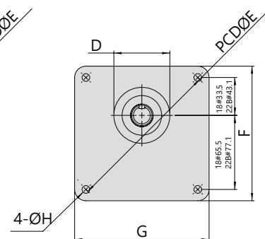
B型法蘭 (框號18、22B用)
